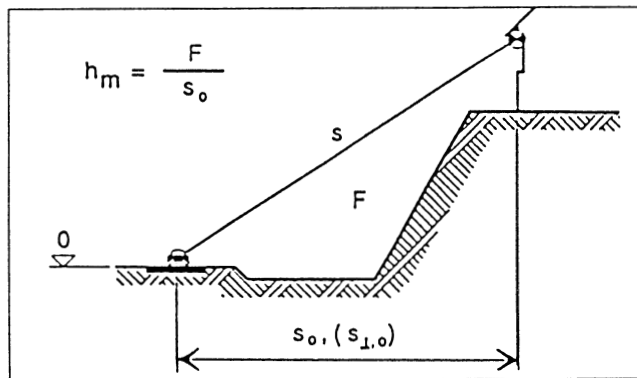
Bild 1: Zur Definition der mittleren Höhe h_m
