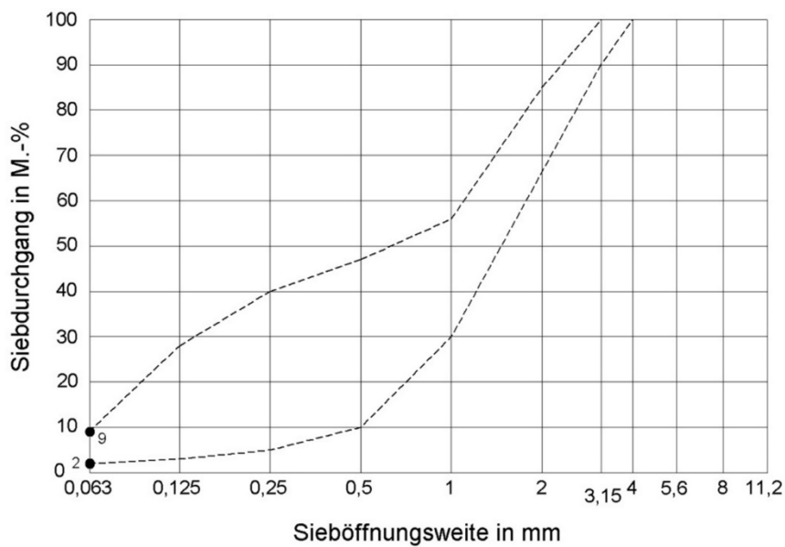
Bild 12: Empfohlener Sieblinienbereich für ungebundenes Fugenmaterial 0/3, welches filterstabil zu einem Bettungsmaterial 0/5 gemäß M FP ist
